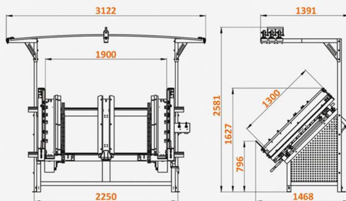
Mått av Pneumatico PT-1900 bordet i mm
